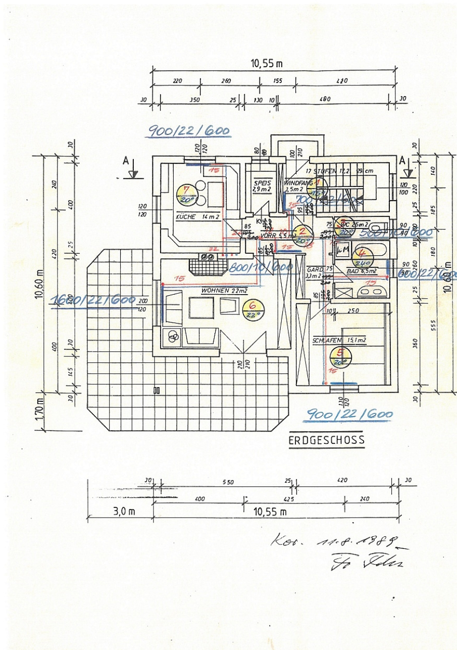
150m² Einfamilienwohnhaus in Klagenfurt
