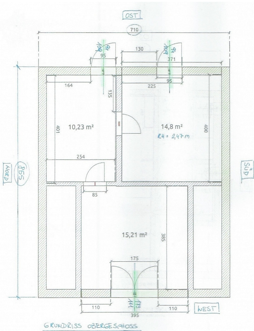
Grundriss Obergeschoss
