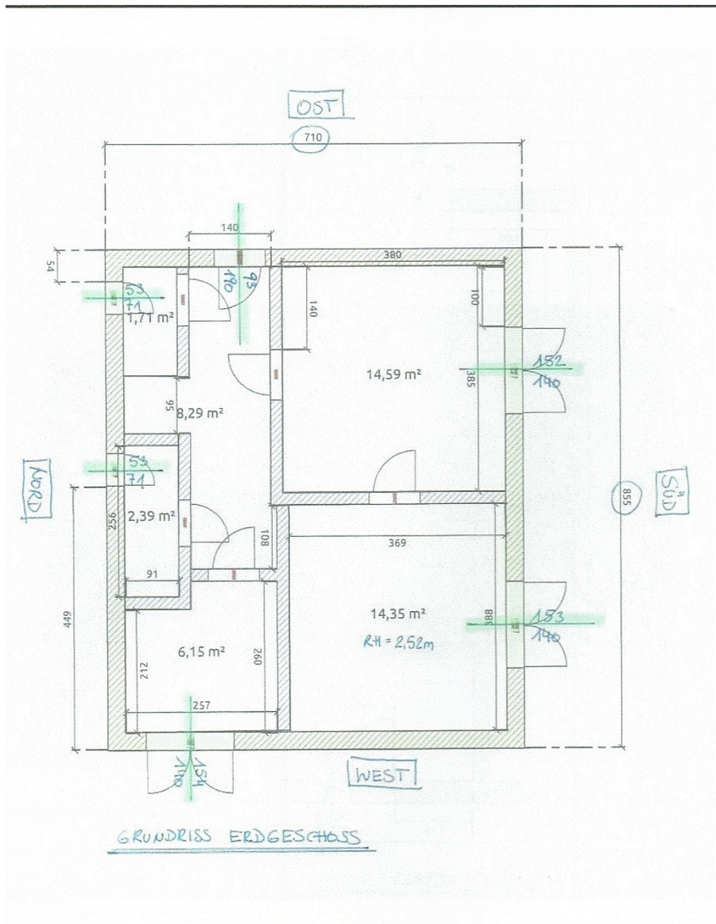
Grundriss Erdgeschoss
